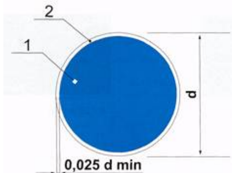
Рисунок 3 - Основа цветографического изображения и соотношение размеров предписывающих знаков безопасности
